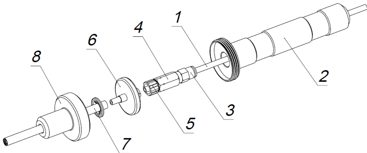
Рис. 1.3. Схема пробоотборника
